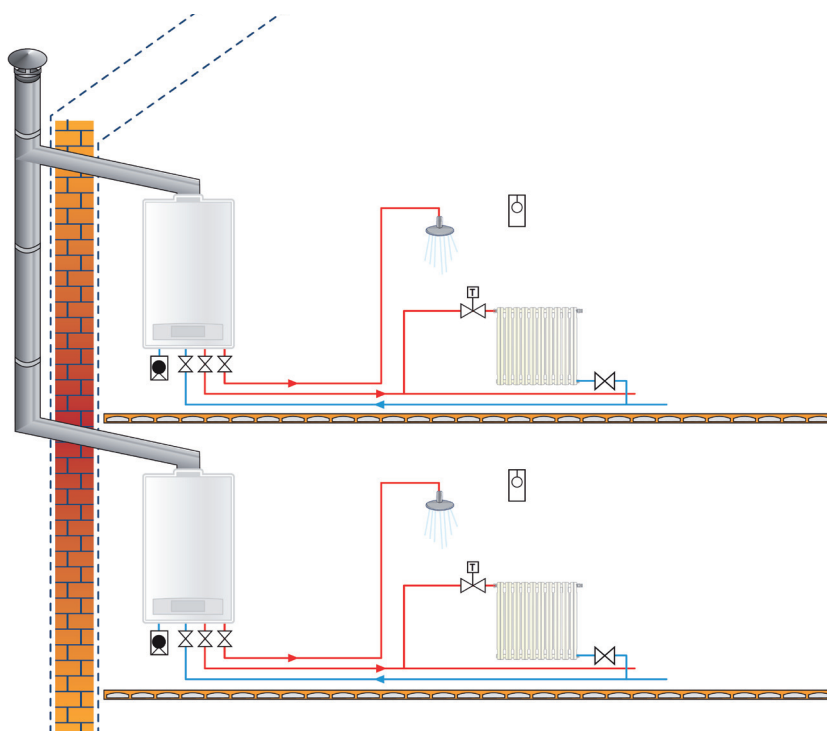
Fig. 2.1 Instalación individual
